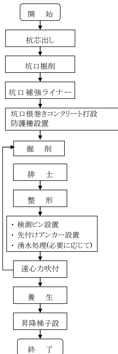
図1.3 深礎工の施工フロー
