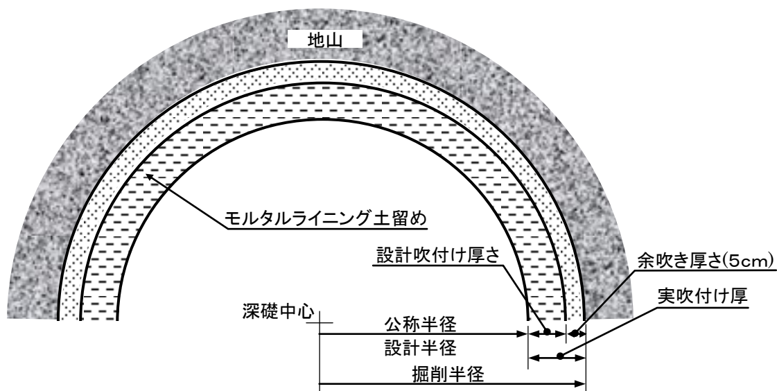
図3. 2 各種寸法(平面図)
