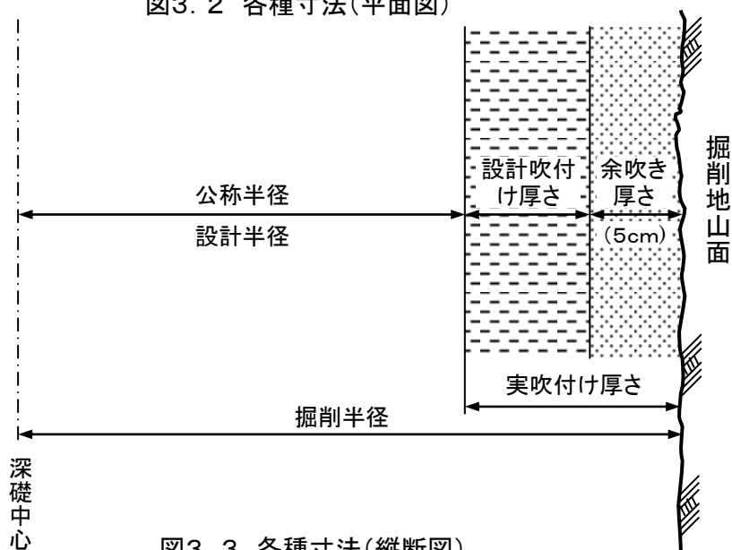
図3. 3 各種寸法(縦断図)
